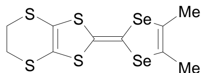
DMET
