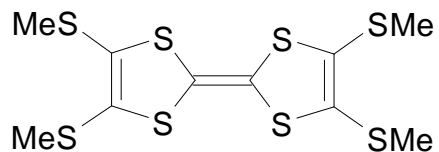
TTM-TTF
