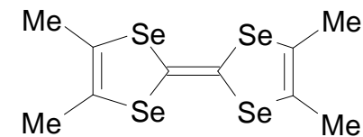
TMTSF
