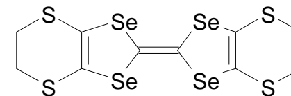
BEDT-TSF (BETS)
