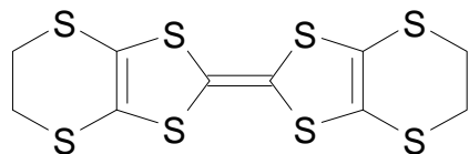
BEDT-TTF (ET)
