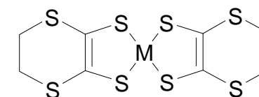
M(dddt) 2 (M=Ni, Pt, Au)
